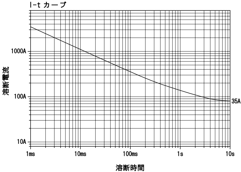
上記の I-t カーブは当社特定試験条件下の実測値の平均をプロットした参考値であり、保証値ではありません
