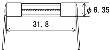
リード線径: \phi 0.8
