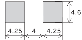
リフローはんだランドパターン (参考寸法)
